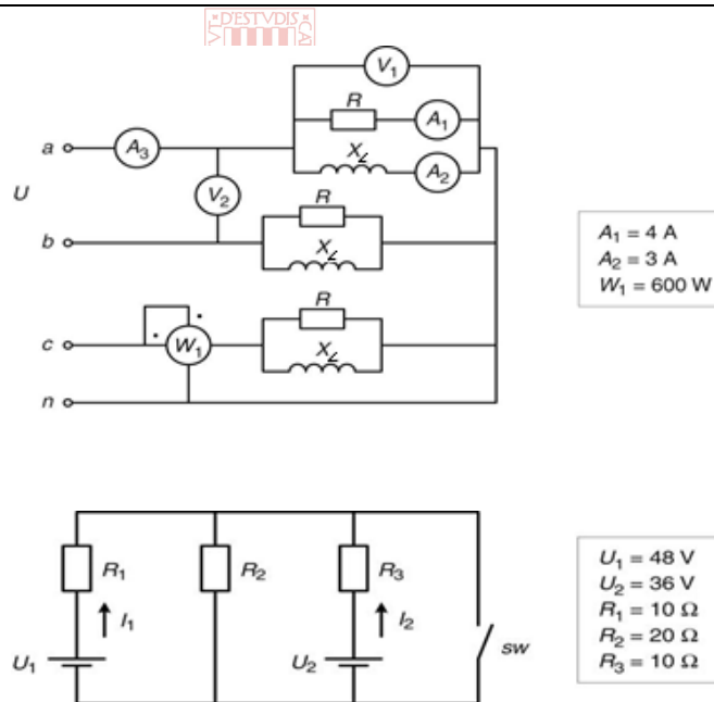
FIGURA 6. Mostra d'esquemes de circuits elèctrics amb símbols associats
