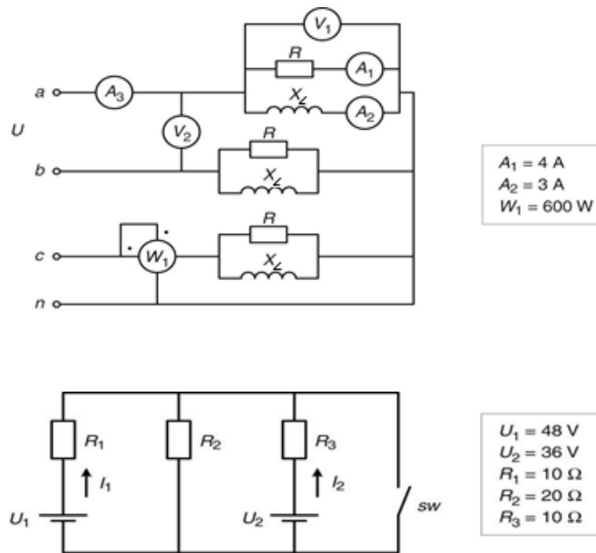
FIGURA 6. Mostra d'esquemes de circuits elèctrics amb símbols associats
